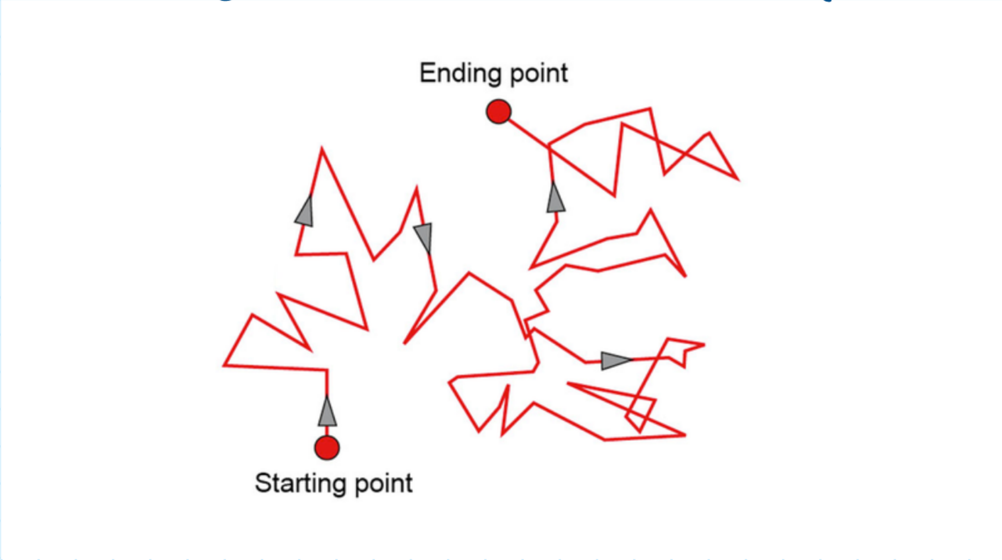
Lëvizja kaotike - Braun'i.
