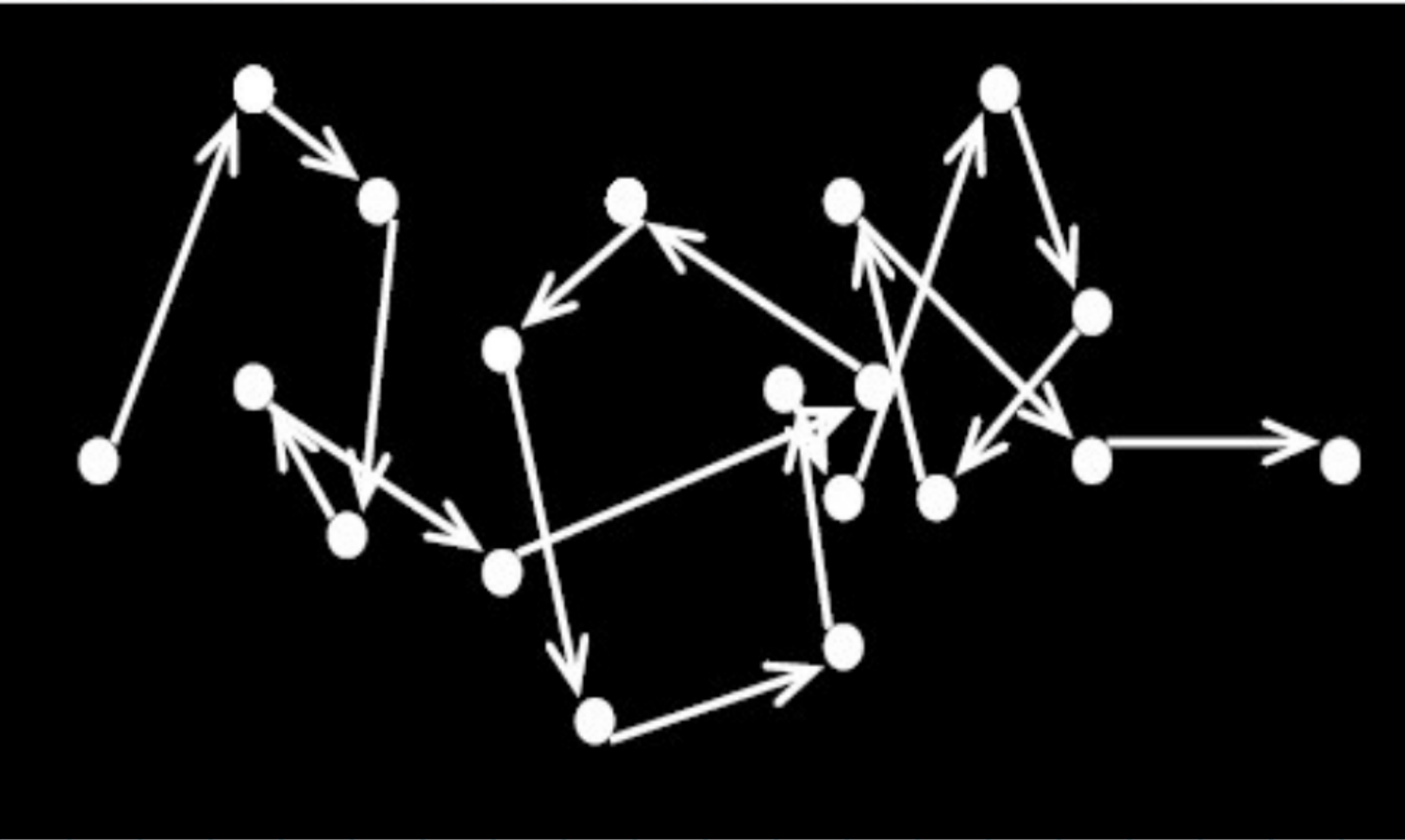
Lëvizja kaotike - Braun'i.
